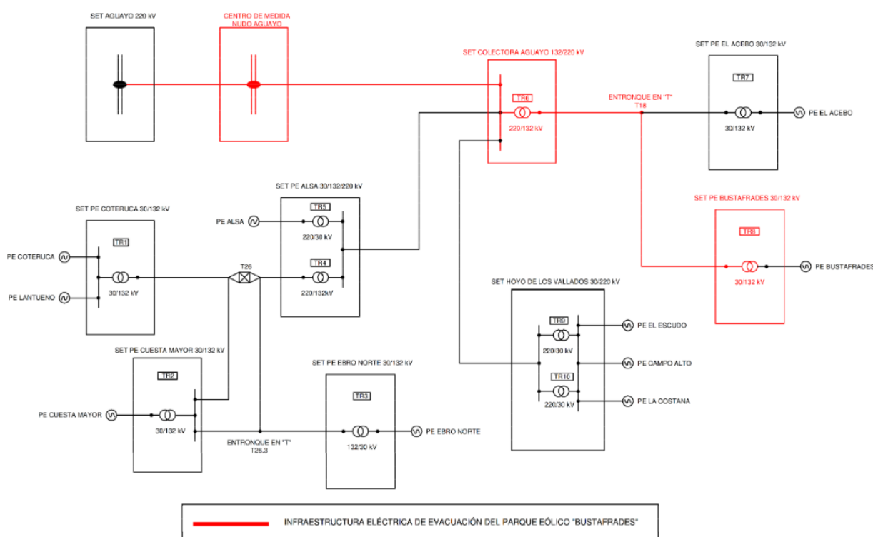
Esquema de parques eólicos interconectados, Pag. 4 del Proyecto LAT, todos ellos promovidos por GCP.
